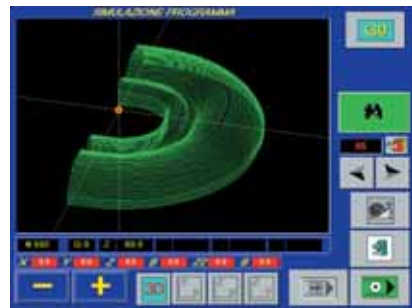
Simulazione di profilo da ottenere con fresa a candela Simulation of a profile to be obtained by shaping tool
